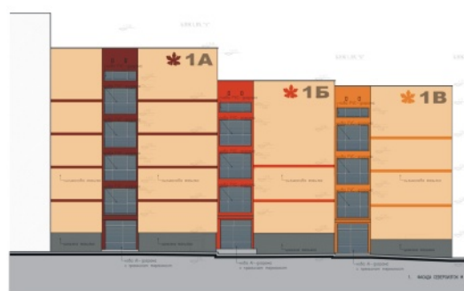
Фасада Блок 1
